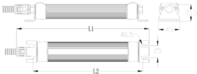
Abmessungen M9SL (in mm)
