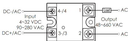
Anschlußplan:
