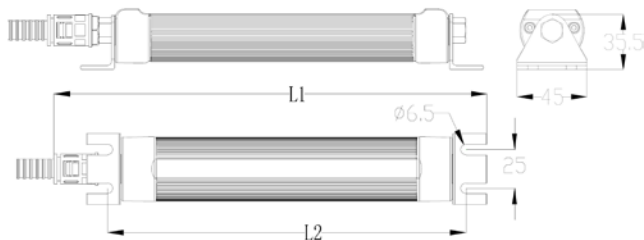
Abmessungen M9SL (in mm)
