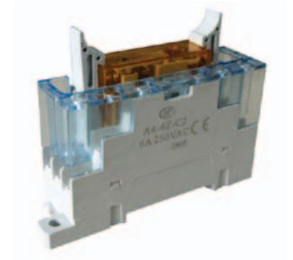
Sockel A4-4Z-C2
