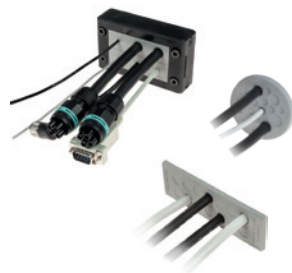
Kabeldurchführungssysteme für nicht- oder für vorkonfektionierte Kabel
