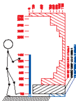
Sicherheitsabstand in einer Höhe von 1 400 mm
